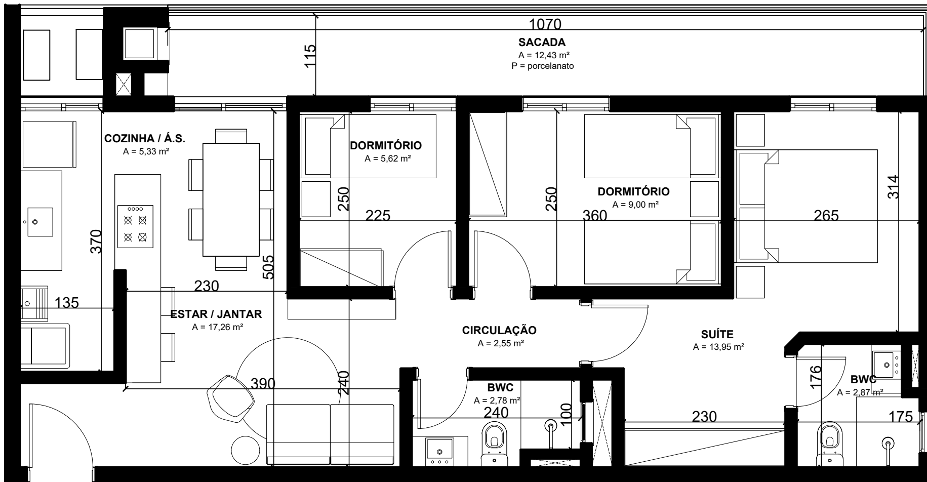
GOLDEN BEACH PLANTA BAIXA FINAIS 01 - 05 ÁREA - 86,95m 2
